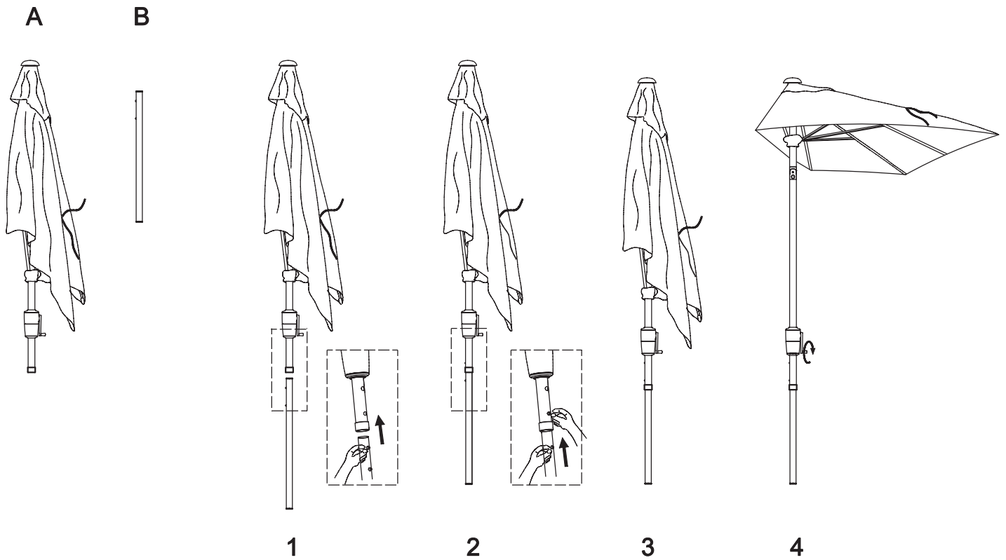
Abbildung 1 und 2: Stock mit 2 Metallknöpfen zur Höhenverstellung um 10 cm
